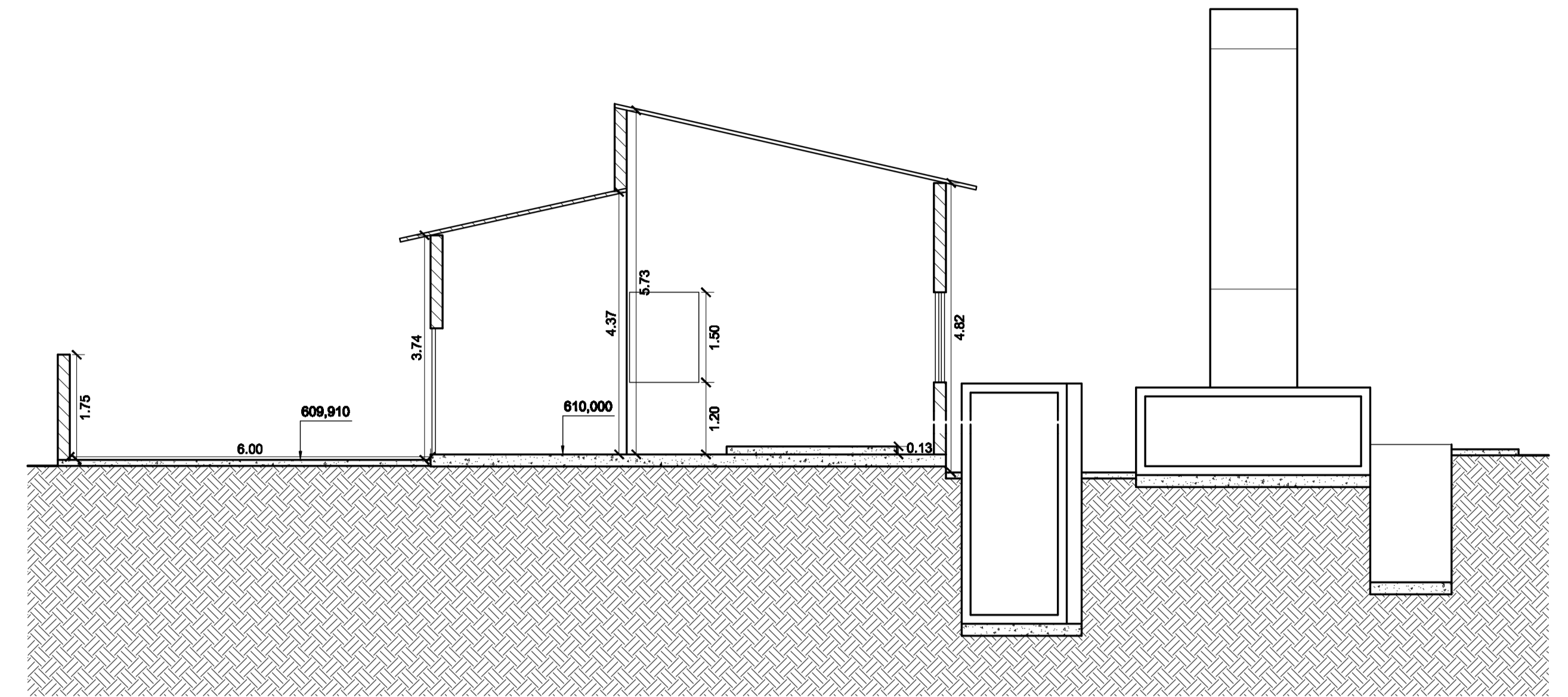
CORTE B.B. ESCALA 1:75
