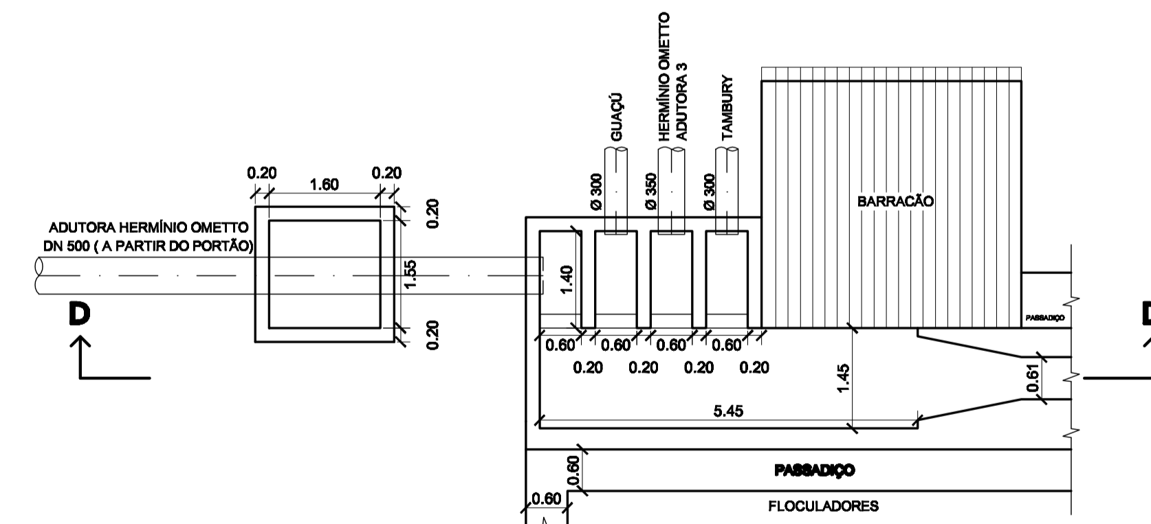
ENTRADA ADUTORA PLANTA BAIXA ESCALA 1:75
